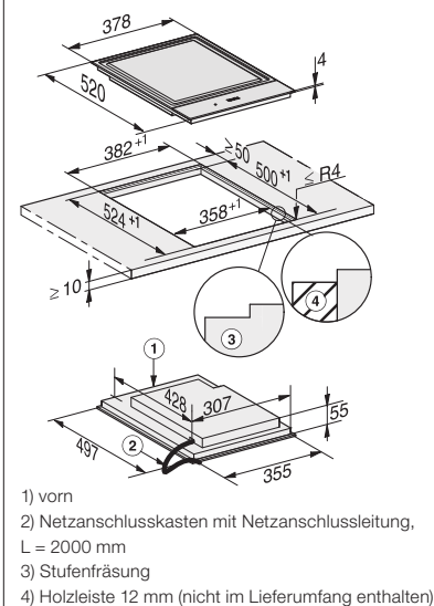
flächenbündiger Einbau
