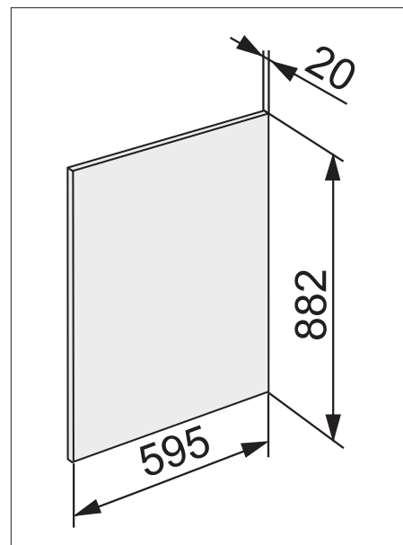
Nachkaufbares Zubehör KEDF 30088 Edelstahl-Frontverkleidung
